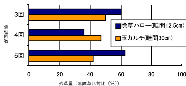
図3 春まき小麦における機械除草効果 (年次(2007～2010)および設定仕様平均)
